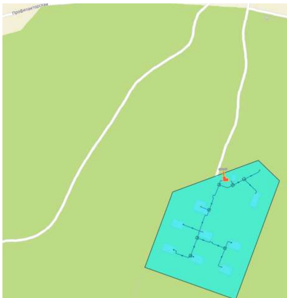
Рисунок 1.31 – Зона действия котельной интернат №66
