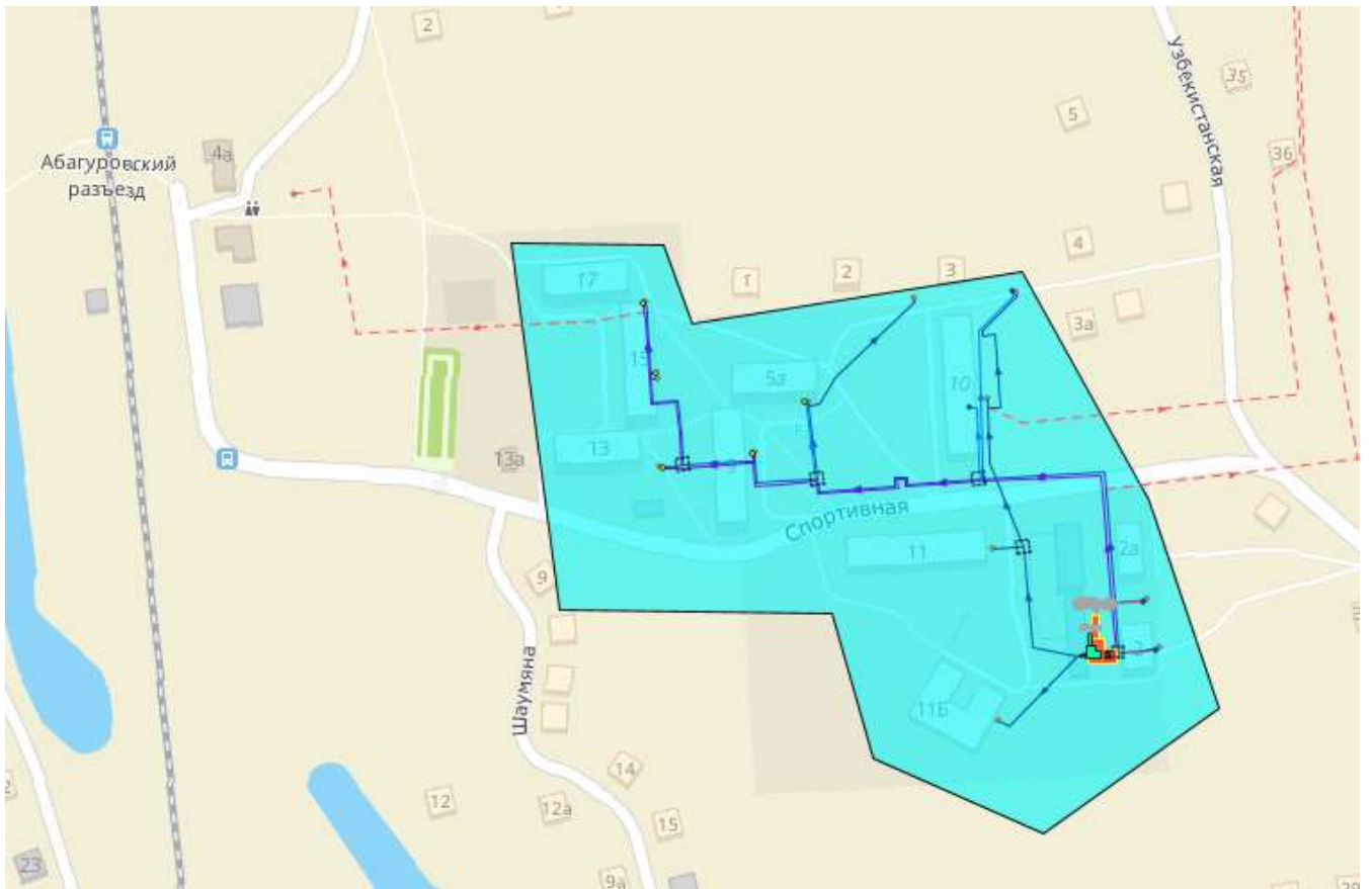
Рисунок 1.23 – Зона действия котельной Разъезд Абагуровский 2
