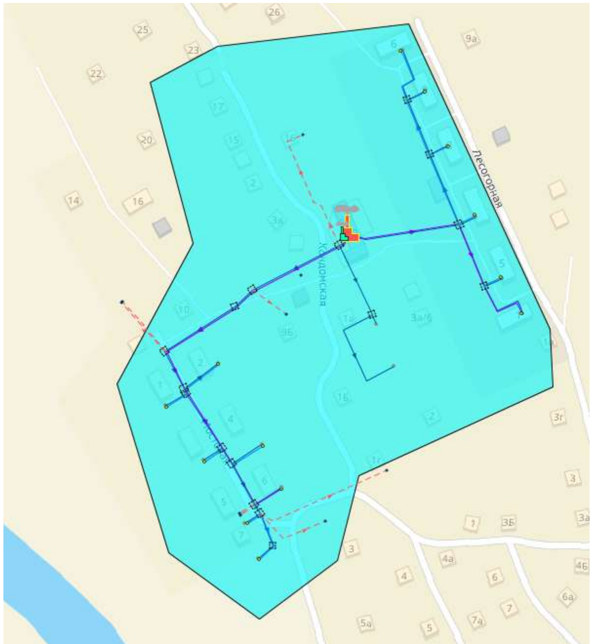
Рисунок 1.22 – Зона действия котельной Разъезд Абагуровский 1
