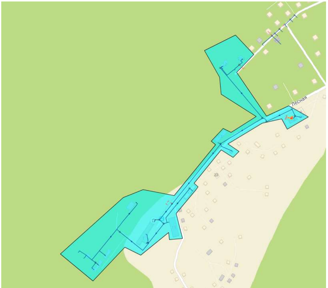
Рисунок 1.15 – Зона действия котельной Таргай
