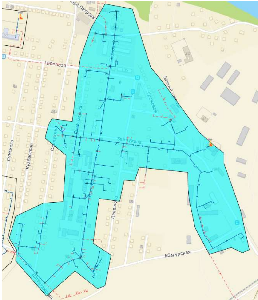
Рисунок 1.16 – Зона действия котельной Абагур-Лесной-1
